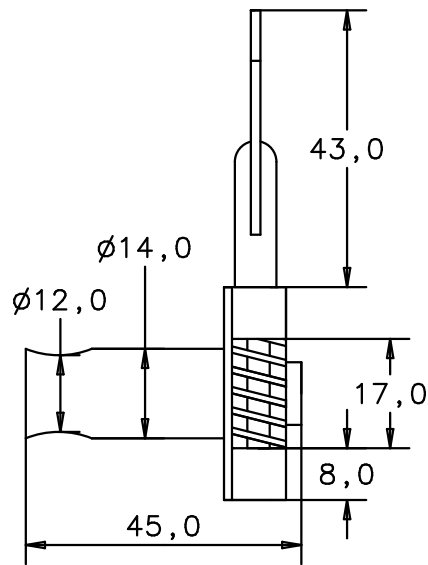
Seitenansicht von links side view left
