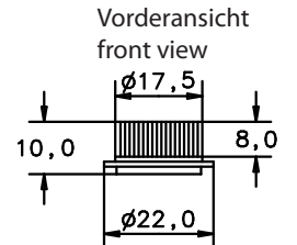
Gegenlager thrust bearing
